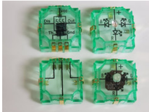
オリジナルブロック例
